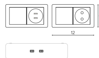
EQ PST1 2x USB + 1x schuko for table top, with 3mt wire 2x USB + 1x schuko per tavolo, con 3mt di cavo 2x USB + 1x schuko pour table, avec 3mt de câble
