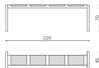
EQ 2204 bench with 4 fixed cushions panca con 4 cuscini fissi banc avec 4 coussins fixes
