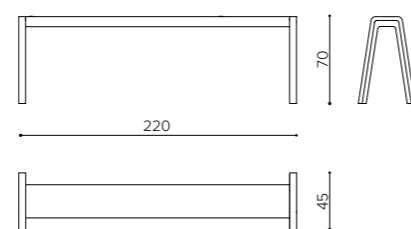
EQ 2200 bench panca banc
