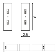
EQ PSB1 4x USB power outlets for bench, with 2mt wire 4x porte ricarica USB per panca, con 2mt di cavo 4x ports de charge USB pour banc, avec 2mt de câble
