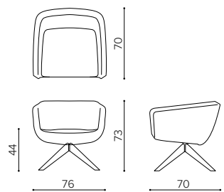
AA 7090 poltrona bassa, base in acciaio low back armchair, steel base
